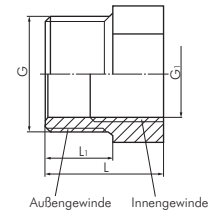
Außengewinde Innengewinde
