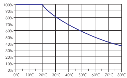
Druck/Temperaturdiagramm PUN-Schläuche
