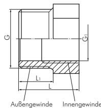
Außengewinde Innengewinde
